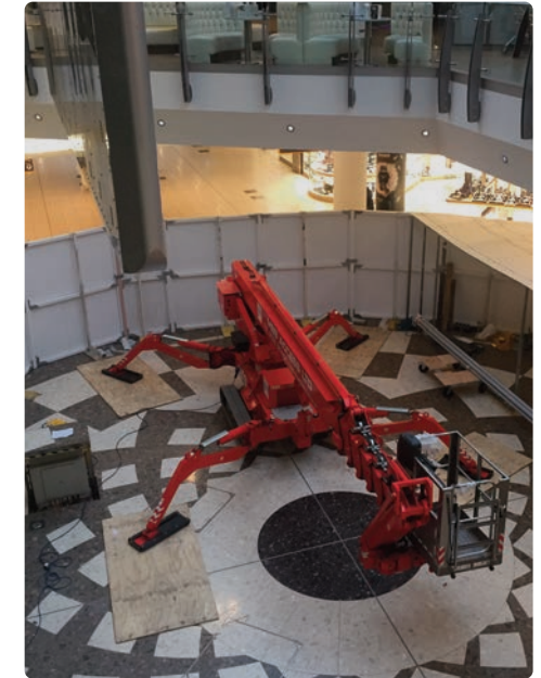
Installatie in een winkelcentrum
