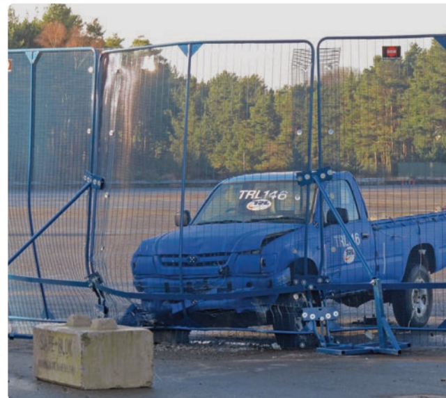
The POLMIL® PAS 68
