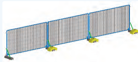
Een opstelling met een Korte schoor en 3 BraceBlok™
